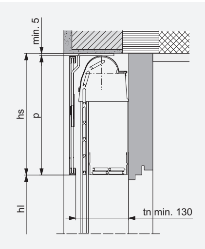
Coupe verticale: Exemple avec lambrequin
