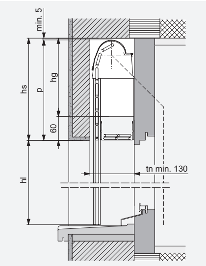
Coupe horizontale: commande par treuil
