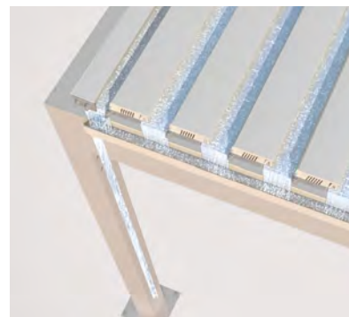
Évacuation de l'eau guidée par un montant
